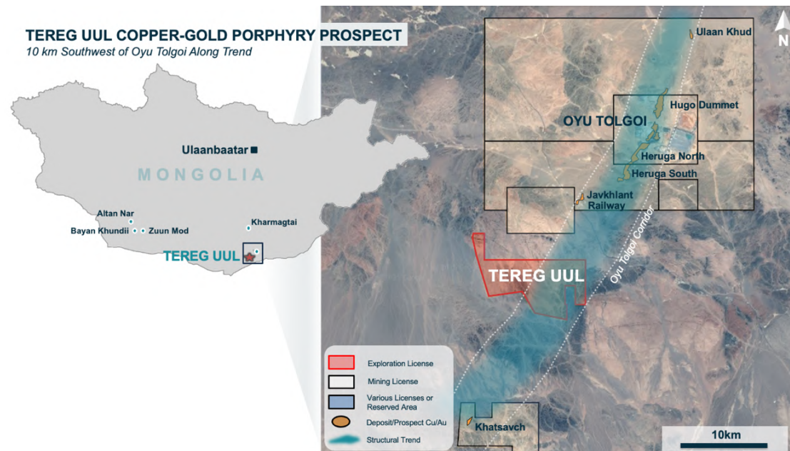
Тэрэг Уул зэс-алтны төсөл – Оюу Толгой дүүрэг, Өмнөговь
