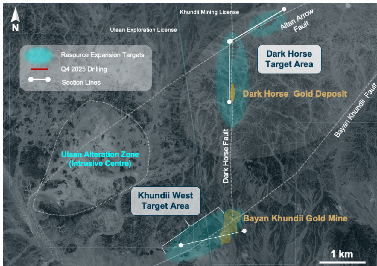
Хөндий алтны хувирлын тренд – Хөндий Эрдсийн Дүүрэг
