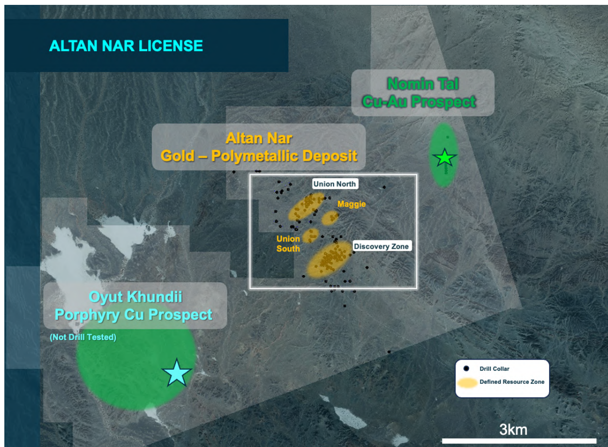
Алтан Нар орд – 5.6 км хүдэржсэн структур
