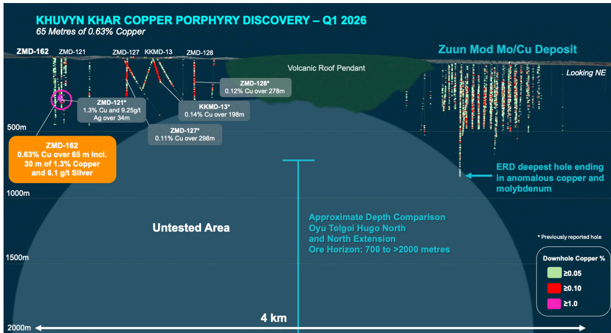
Хөвийн Хар порфирийн систем (Зуун Мод ордыг агуулсан)
